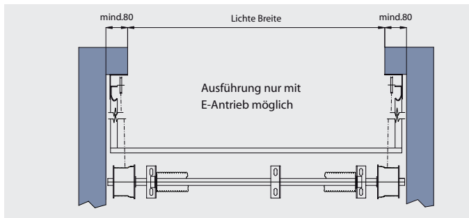
Draufsicht
