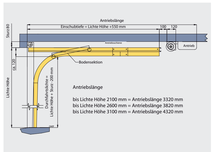
Seitenansicht
